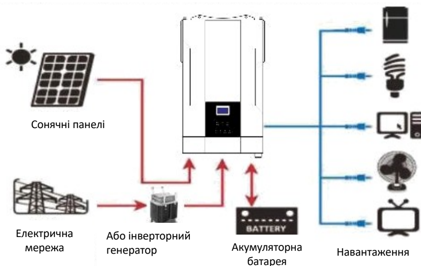
Малюнок 1 Архітектура базової автономної фотоелектричної системи
