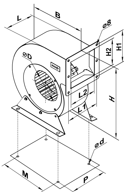
Габаритные размеры и варианты положения корпуса вентилятора ВЦУ
