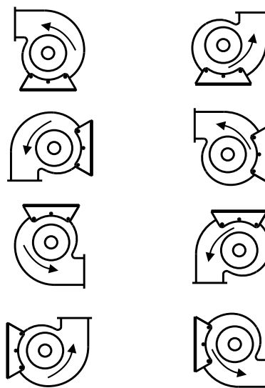
ВОЗМОЖНЫЕ ВАРИАНТЫ ПОЛОЖЕНИЯ КОРПУСА ВЕНТИЛЯТОРА ВЦУ (вид со стороны притока воздуха)
