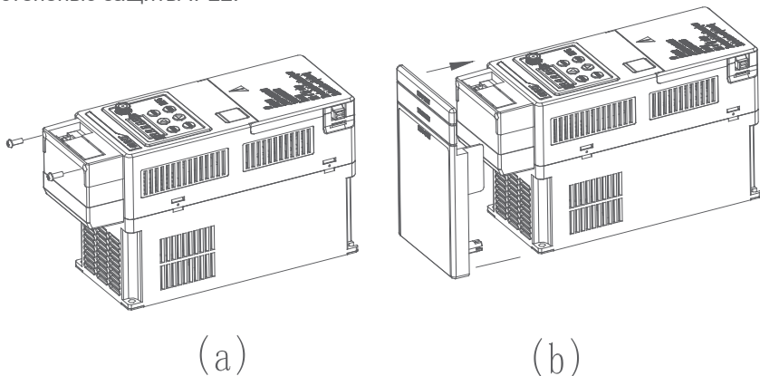
Установка кронштейна и защитной крышки.
