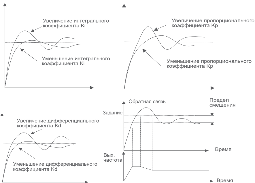
Влияние коэффициентов на характеристики переходного процесса
