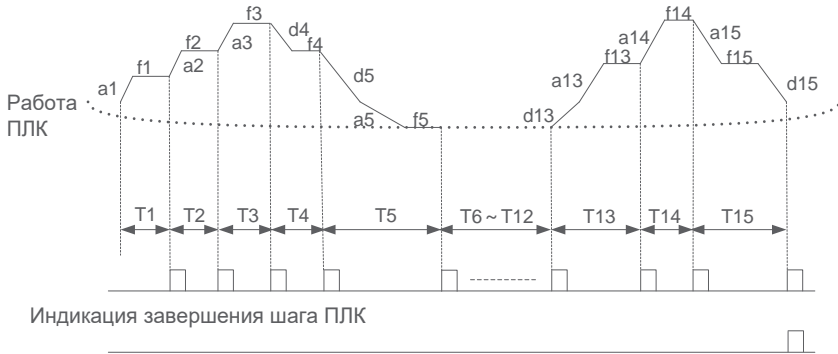
Диаграмма работы ПЛК как источника задания частоты
