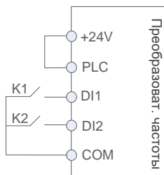
Диаграмма двухпроводного управления, режим 2
