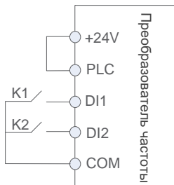
Диаграмма двухпроводного управления, режим 1
